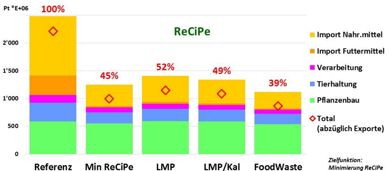
Abbildung 4: Umweltwirkung ReCiPe (Referenz = 100%)
